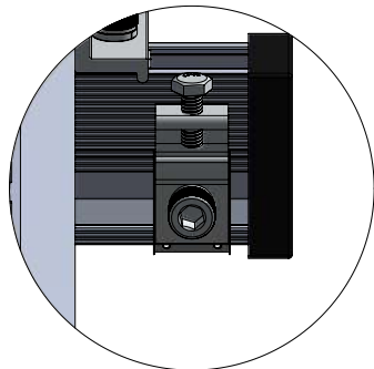
DETALLE G GROUND LUG
