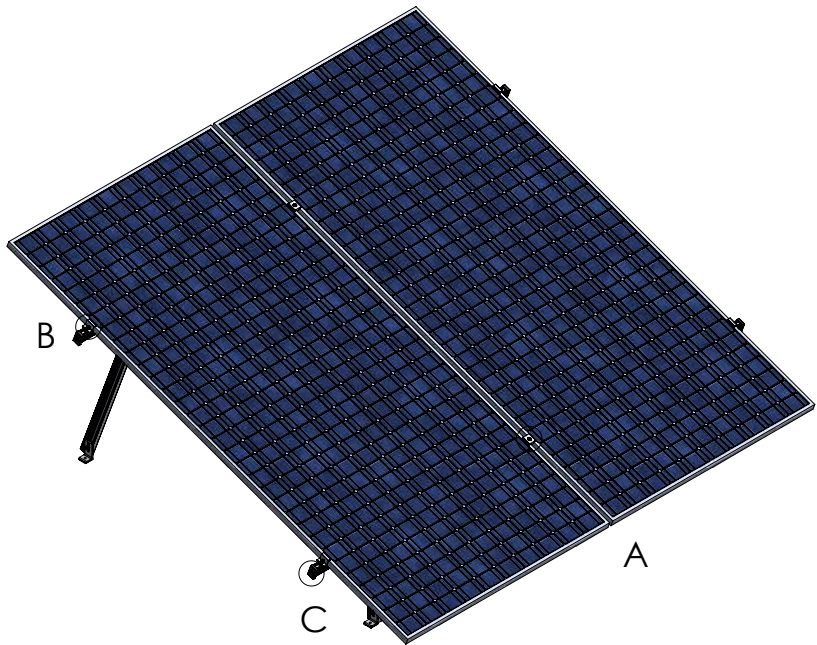
VISTA ISOMETRICA
