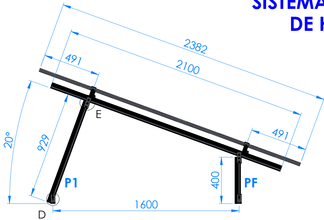
VISTA LATERAL
