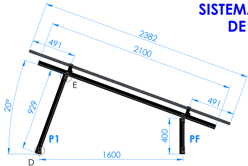
VISTA LATERAL
