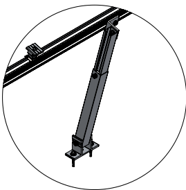
DETALLE B PATA TRASERA AJUSTABLE
