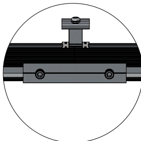
DETALLE F EXTENSIÓN PARA PERFIL RIEL
