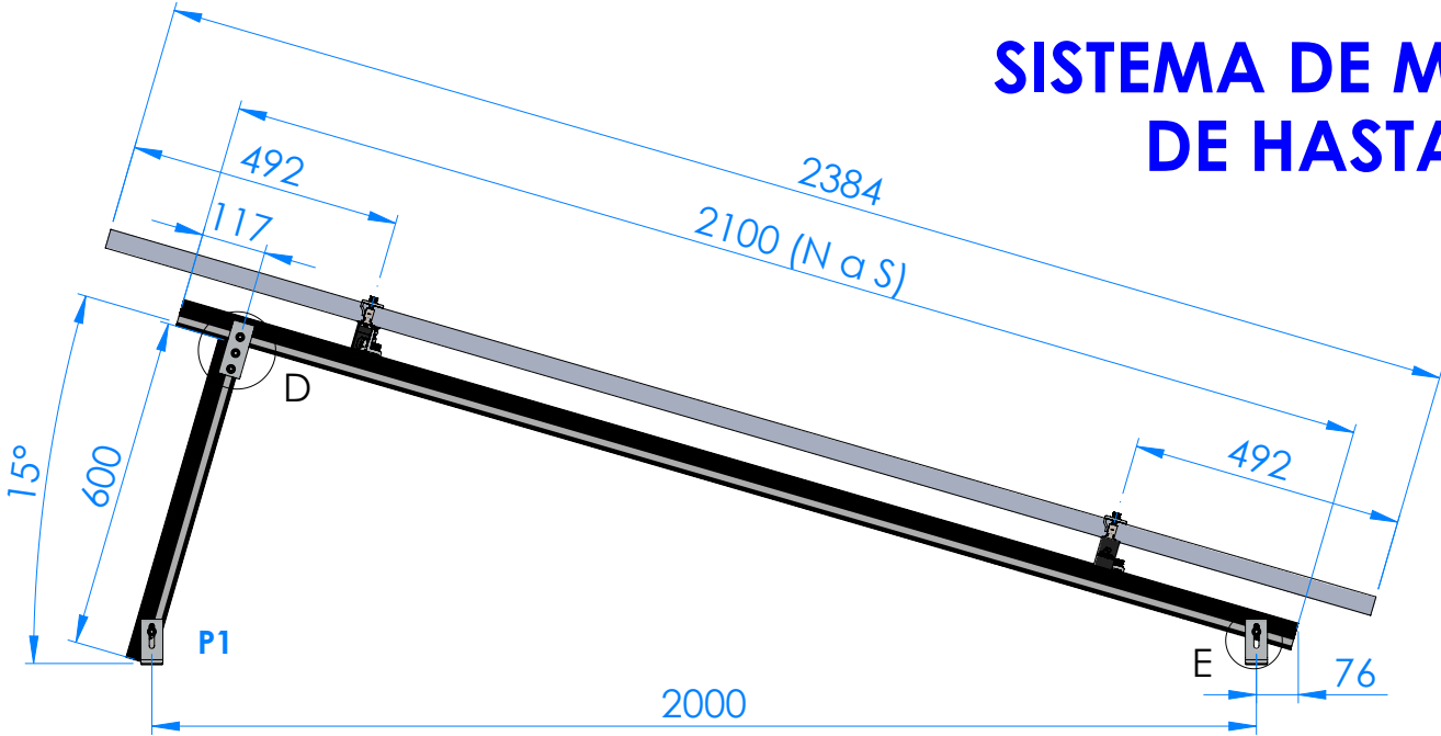
VISTA LATERAL
