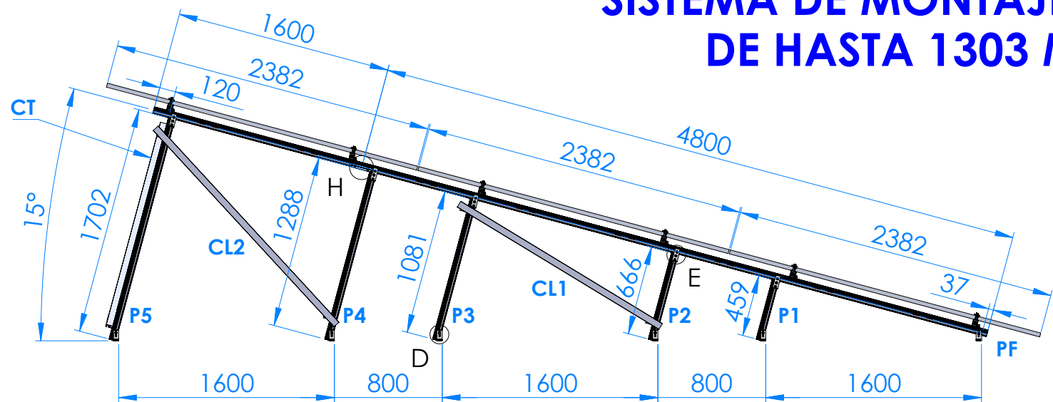
VISTA LATERAL
