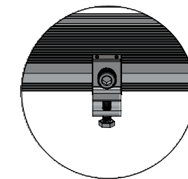
DETALLE E GROUND LUG
