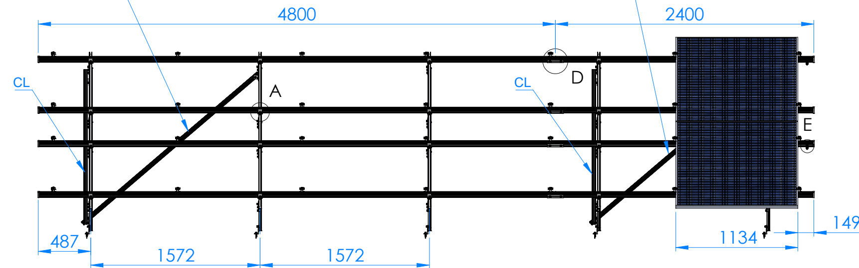
CONTRAVIENTOS TRASEROS (CT)
